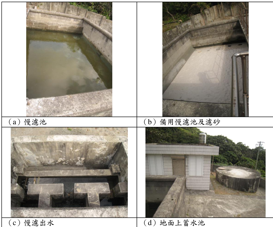
圖 1.2 某簡易自來水場淨水設備（原水→慢濾→出水，可配合自動加氣機操作）
